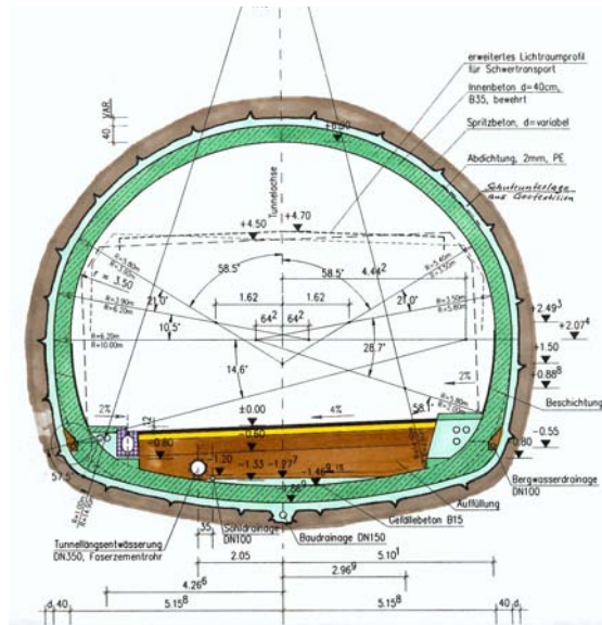
Baggervortrieb im Kalottenquerschnitt
